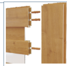
Pevné lepené kolíkové spoje s perodrážkou
